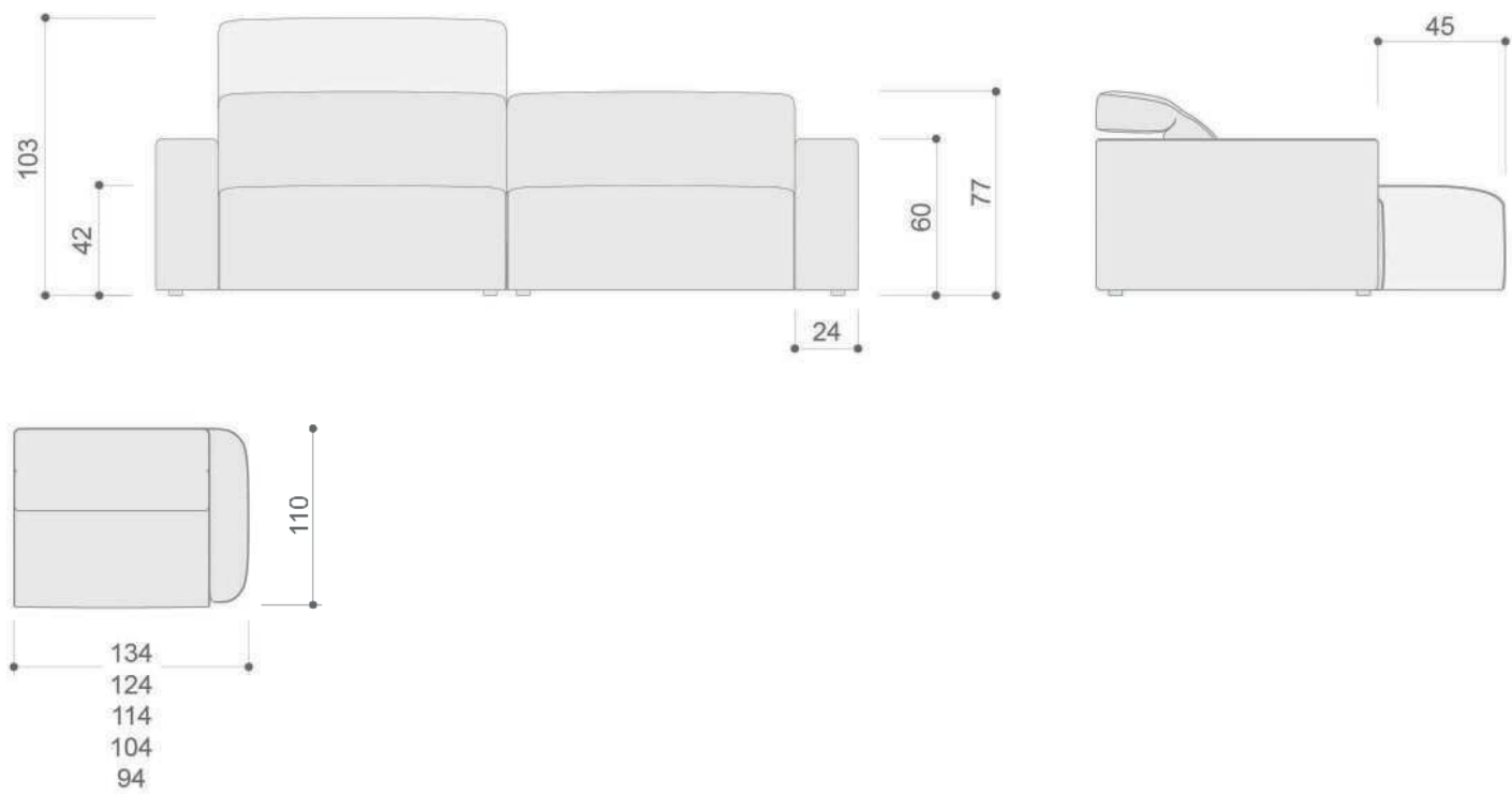
Módulo con 1 brazo
