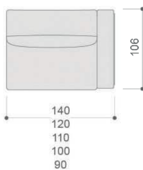
Módulo fijo con 1 brazo
