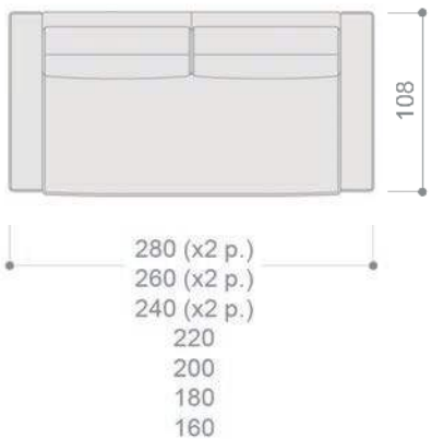
Sofá con 2 brazos/Asiento en 1 pieza
