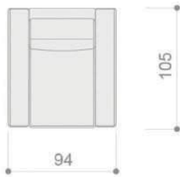
Módulo sin brazos
