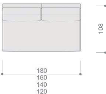
Sofá sin brazos/Asiento en 1 pieza
